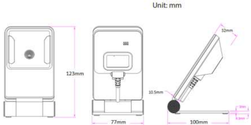
外形寸法 (mm)
